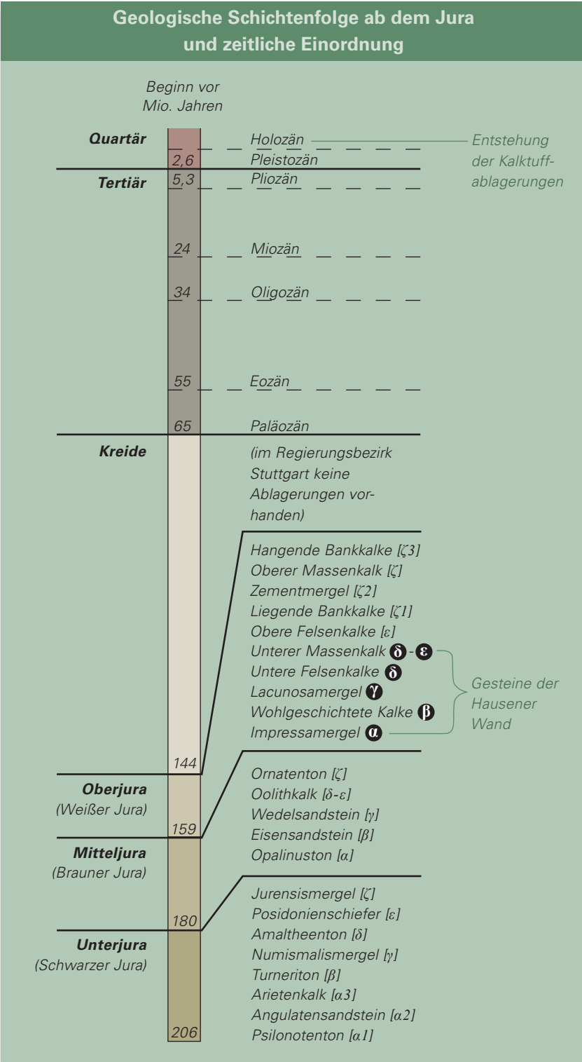
Abb. 18: Geologische Schichtenfolge ab dem Jura und zeitliche Einordnung. Im Projektgebiet Filsalb sind insbesondere die obersten Mitteljuraschichten, der Oberjura und das Holozän (Kalktuffablagerungen) von Bedeutung.
